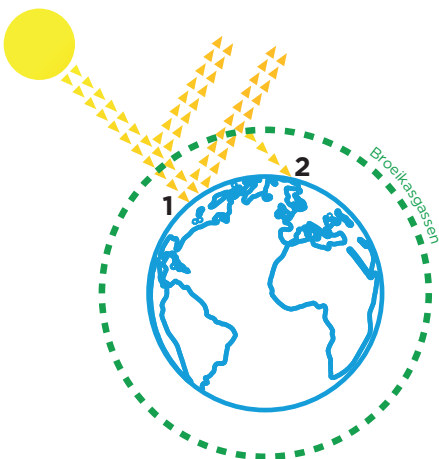
Natuurlijk broeikaseffect
