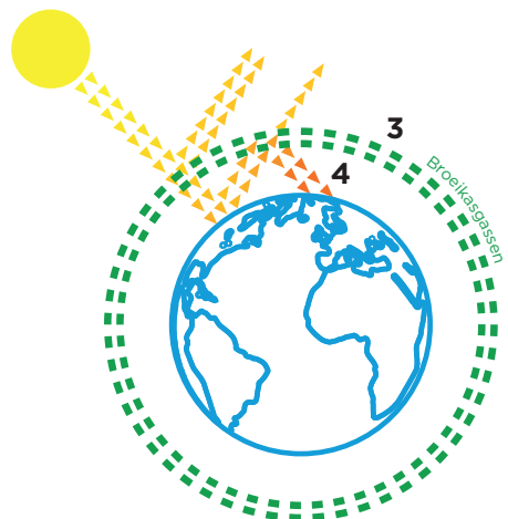
Versterkt broeikaseffect
